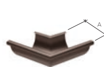
łuk 90° zewnętrzny*
