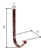
hak metalowy nakrętkiowy grubość haka wynosi 3 mm
