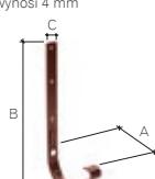
hak met. nakrokwiiowy wzmocniony grubość haka wynosi 4 mm
