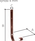
hak met. nakrętkiowy wzmocniony grubość haka wynosi 4 mm
