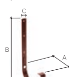
hak metalowy nakrokwiovym grubość haka wynosi 3 mm
